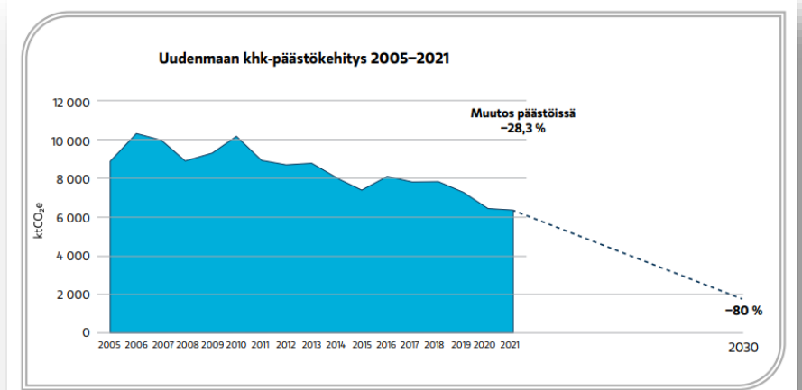
Kuva 3. Uudenmaan kokonaispäästöt ja polku hiilineutraaliuteen vuoteen 2030. Hiilineutraaliuden määritelmänä pidetään yleisesti 80 % päästövähennystä. Loppuosan ajatellaan sitoutuvan hiilineluihin ja kompensoitavan muilla keinoin.
